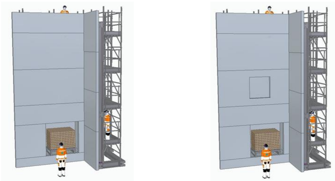
Fig.1 – Schema 3D dell'impianto di prova “large exposure fire test”
